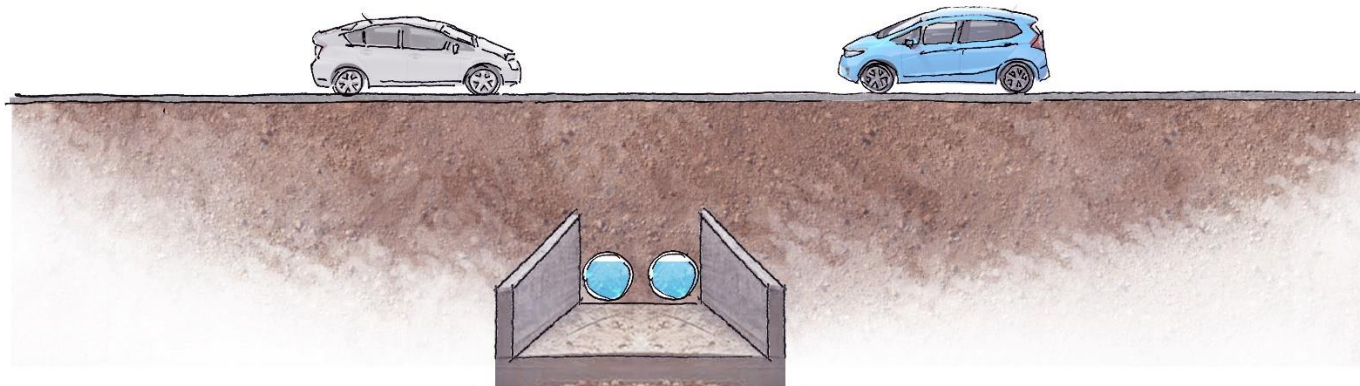
חתך מצב קיים
