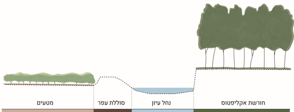
חתך מצב קיים
